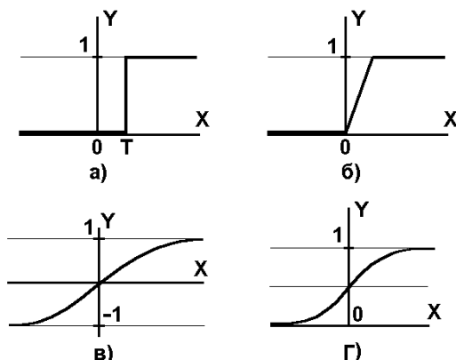
Рис. 2. а) функция единичного скачка; б) линейный порог (гистерезис); в) сигмоид – гиперболический тангенс; г) сигмоид – формула (3)
