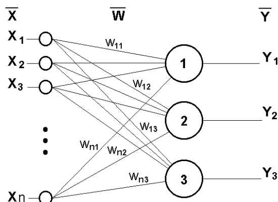
Рис.3. Однослойный перцептрон
