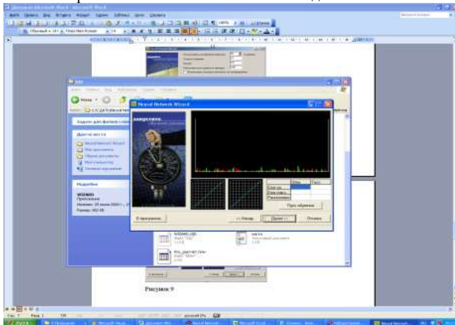
Рисунок 2.6 – Обучение системы
