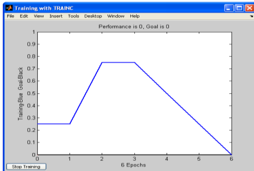
Рисунок 4.9 – Кривая обучения
