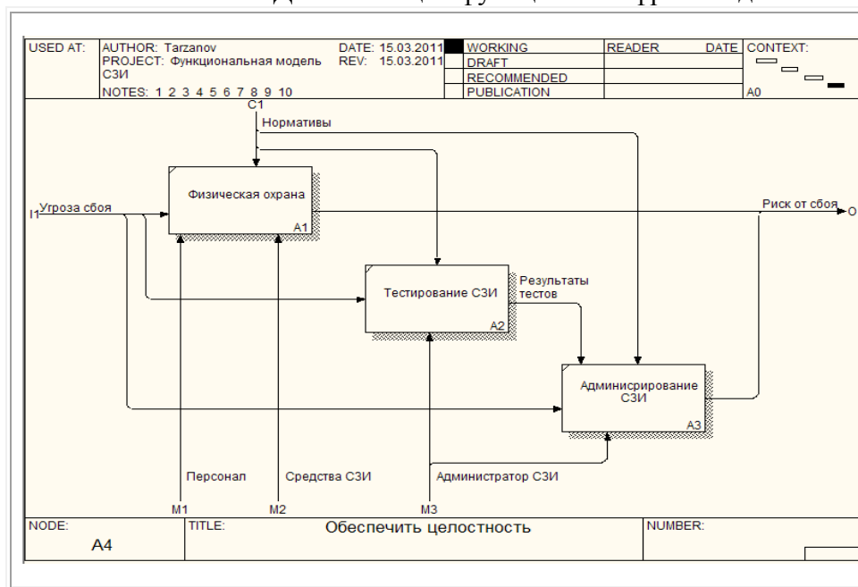
Рис. 2.7. Декомпозиция функции «Обеспечить целостность»
