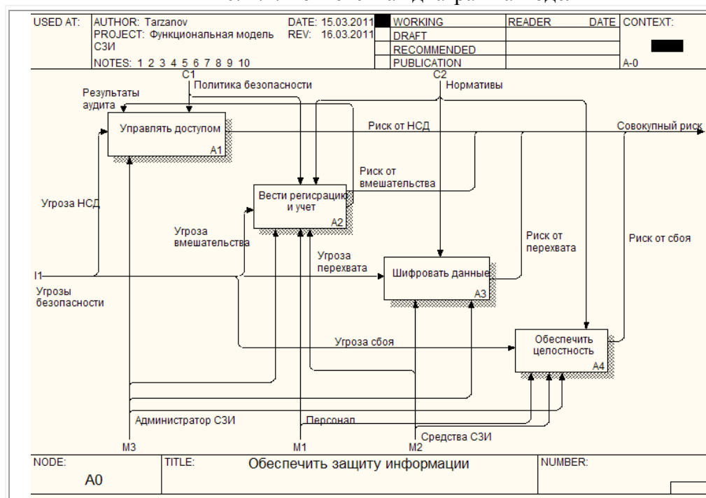
Рис. 2.3. Декомпозиция основной функции
